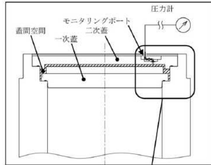
<蓋部断面図>
