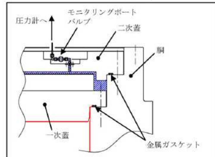
<蓋部詳細図>
