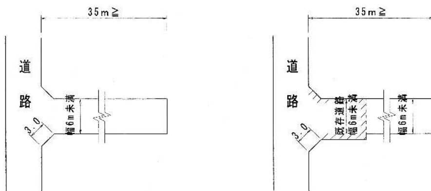
参考図－6 道路の回転広場等
