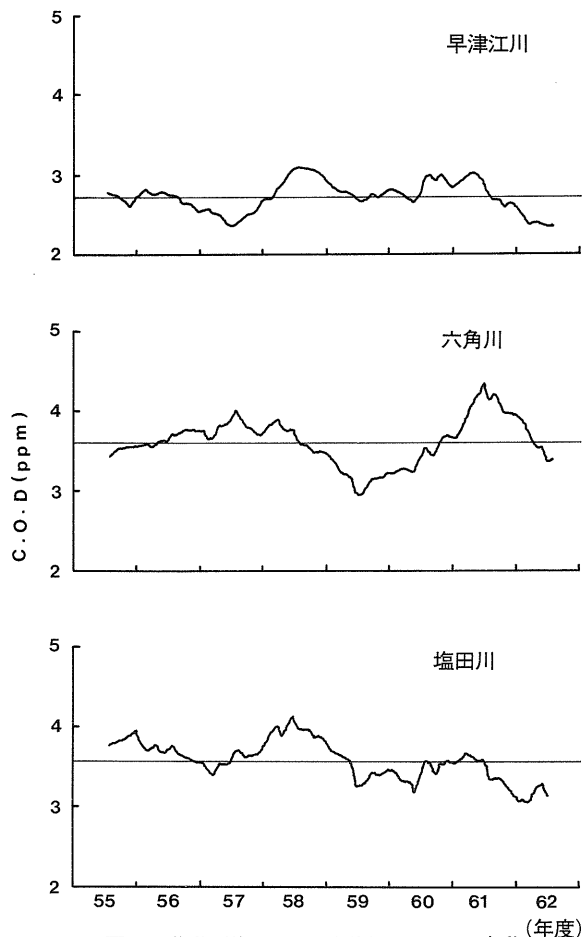
図6 移動平均による3河川のCODの変動 実線は8ヶ年平均値
